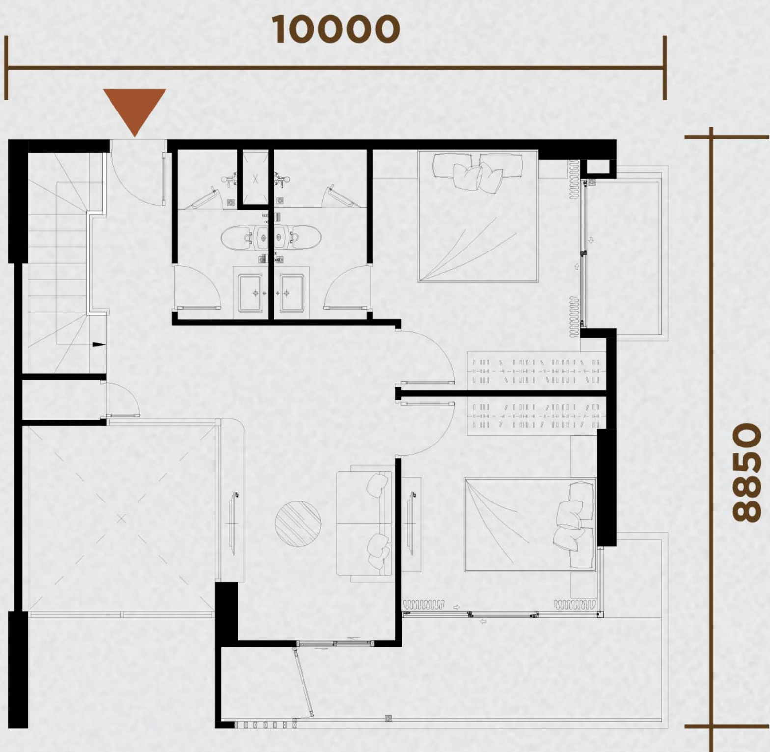
DT sử dụng: 68.86m 2 DT xây dựng: 72.59m 2 Mặt bằng tầng 2
