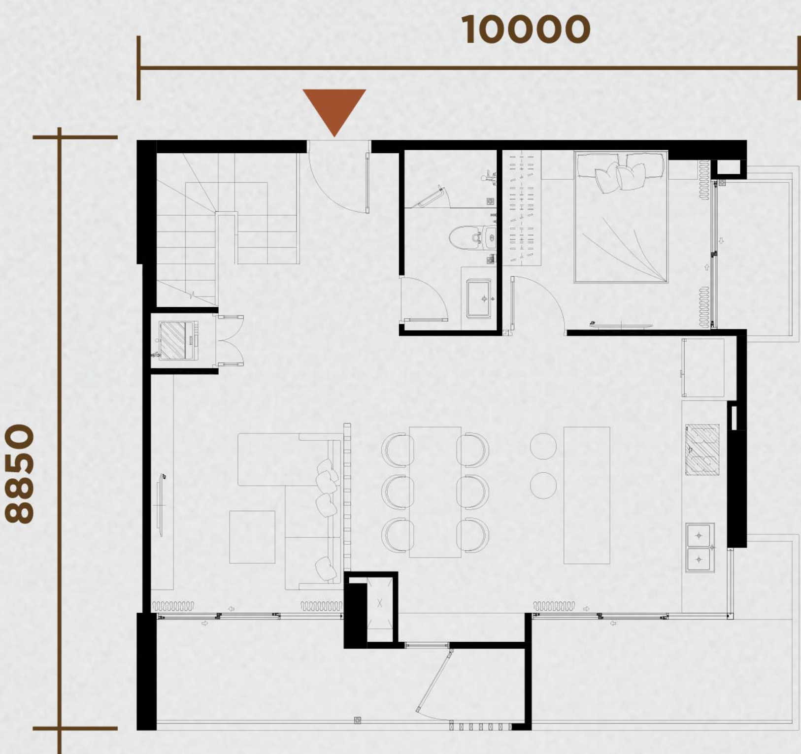
DT sử dụng: 82.08m 2 DT xây dựng: 86.80m 2 Mặt bằng tầng 1
